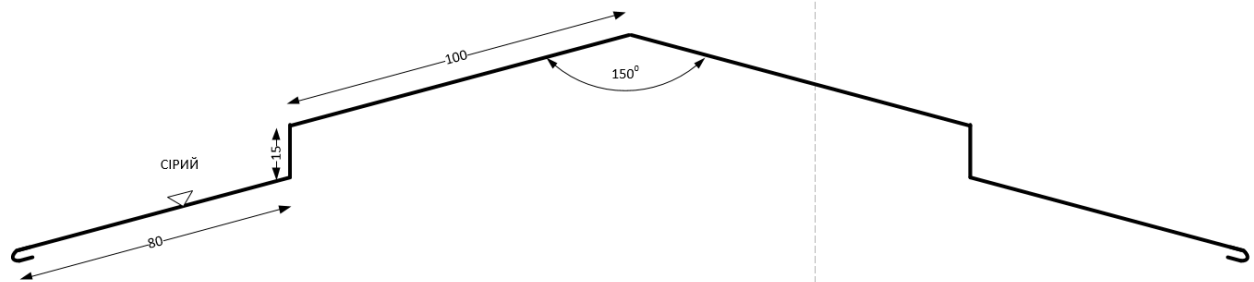
4 Конькова планка зовнішня
