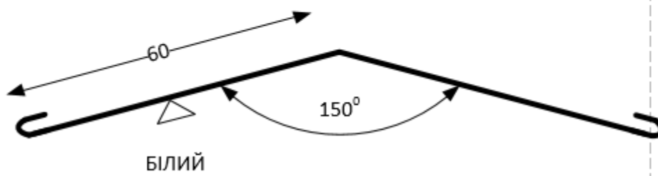
5 Конькова планка внутрішня
