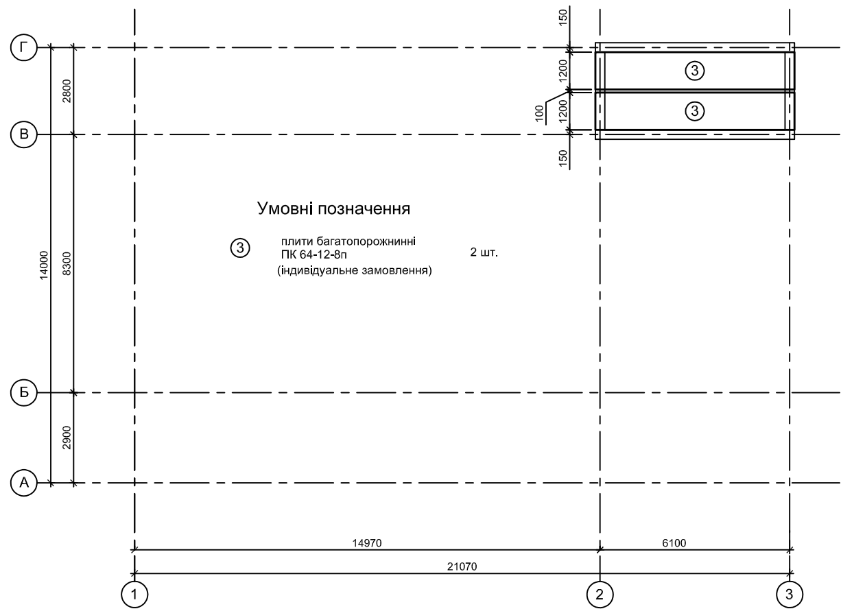
Схема влаштування покриття сходової клітини
