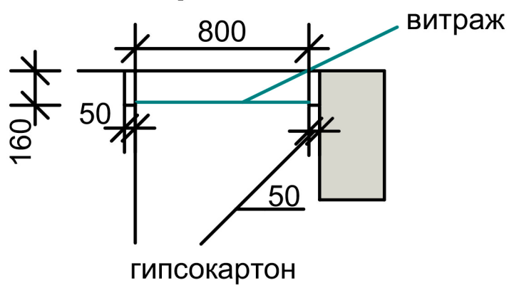
Разрез 2-2
