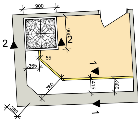
План потолок сан.узел 2й эт
