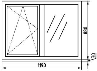
Кол-во 1шт. Стеклопакет 4i 10Ар 4 10Ар 4i
