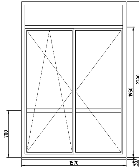
Стеклопакет 4i 10Ар 4 10Ар 4i
