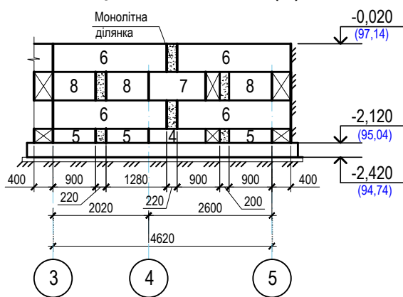
Розгортка по осі В (Г)
