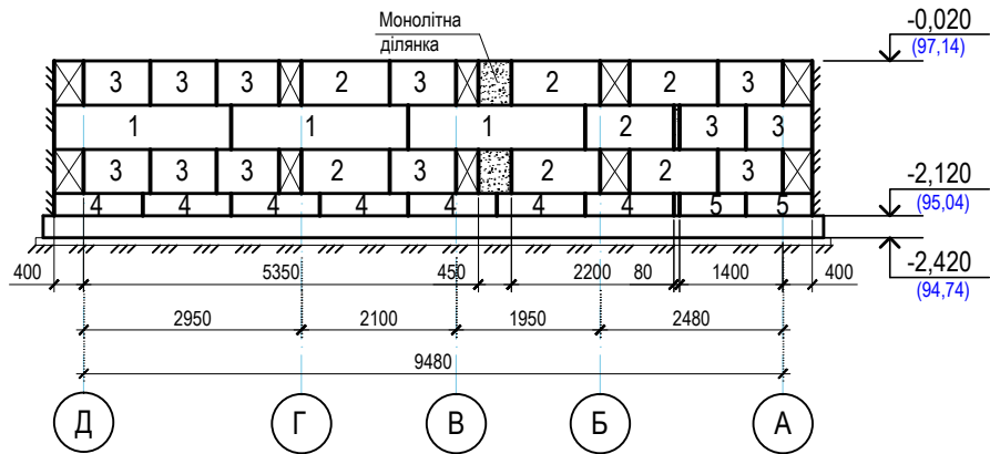
Розгортка по осі 5
