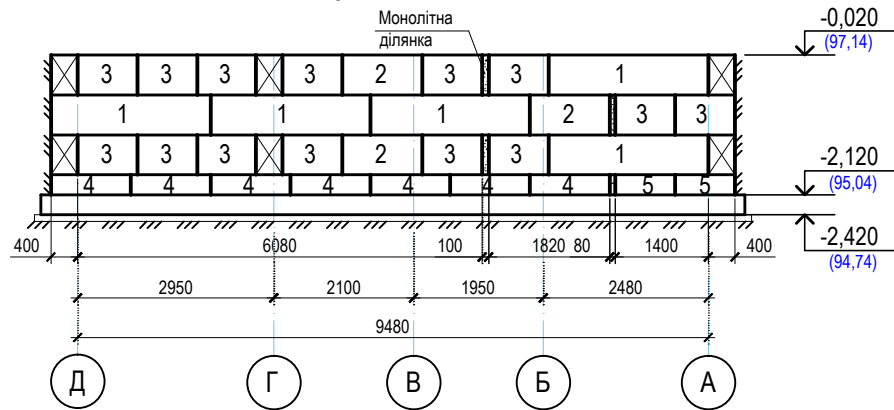
Розгортка по осі 3
