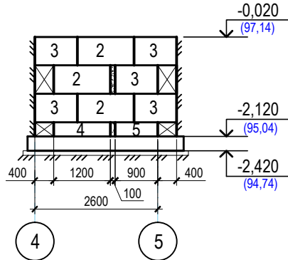
Розгортка по осі Д
