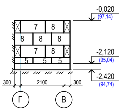
Розгортка блоків між осями 4 - 5
