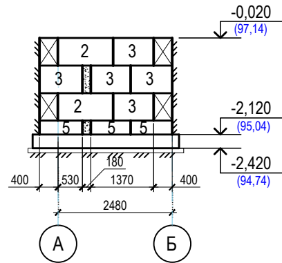
Розгортка по осі 4
