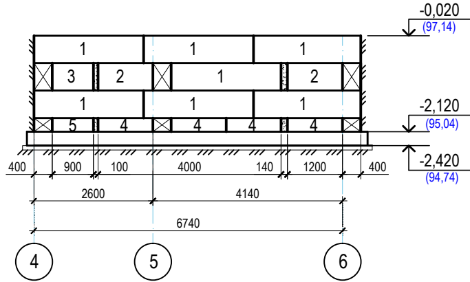
Розгортка по осі Б
